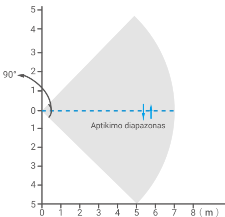
2 pav. Aptikimo diapazono vaizdas iš viršaus
