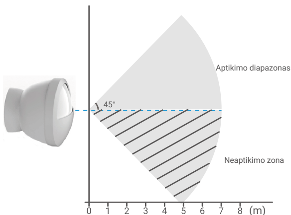
2 pav. Aptikimo diapazono vaizdas iš viršaus
