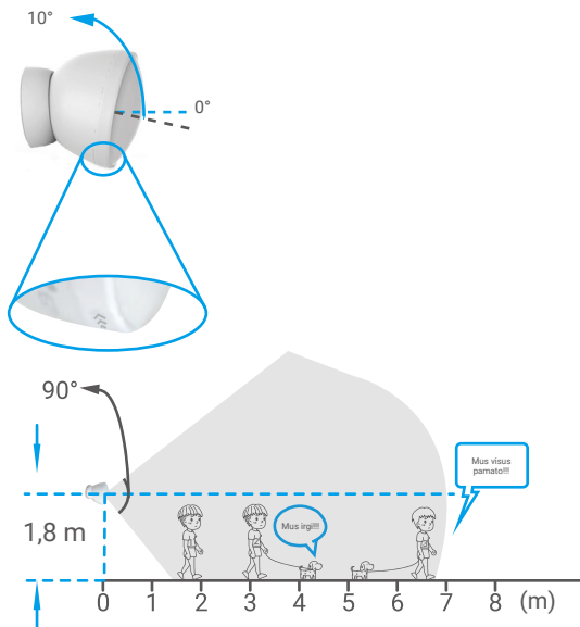
1 pav. Aptikimo diapazono vaizdas iš šono
